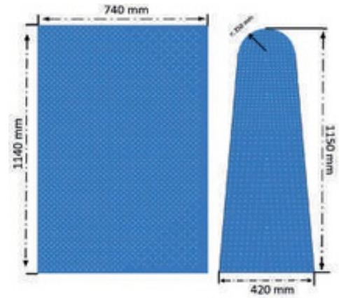
GENİŞ VAKUMLU MİNİ ÜTÜ KOYMA YERLİ PASKALA WIDE IRONING TABLE WITHIN VACUUM (SEAT FOR MINI BOILER) ПРЯМОУГОЛЬНЫЙ УТЮЖИЛЬНЫЙ СТОЛ С ВАКУУМНОЙ ВЫТЯЖКОЙ И ГЛАДИЛЬНЫМ РУКАВОМ
